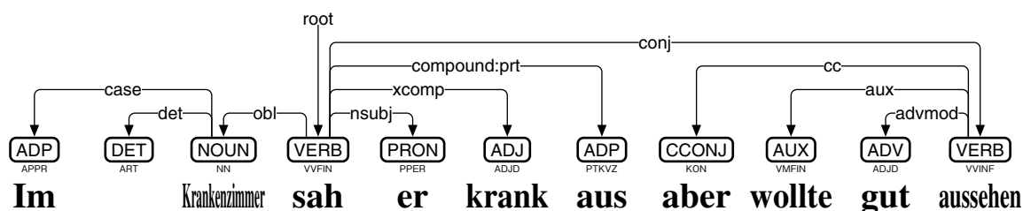
図 55: Trankit によるドイツ語の係り受け解析
