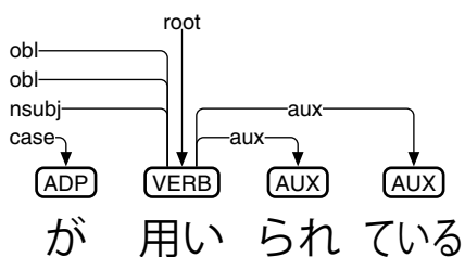
図 34: roberta-base-japanese-luw-upos による日本語係り受け解析 (国語研長単位)
