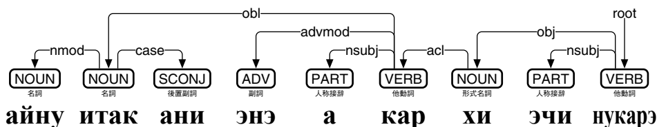
図 175: deberta-base-ainu-upos によるアイヌ語(キリル文字)の係り受け解析
