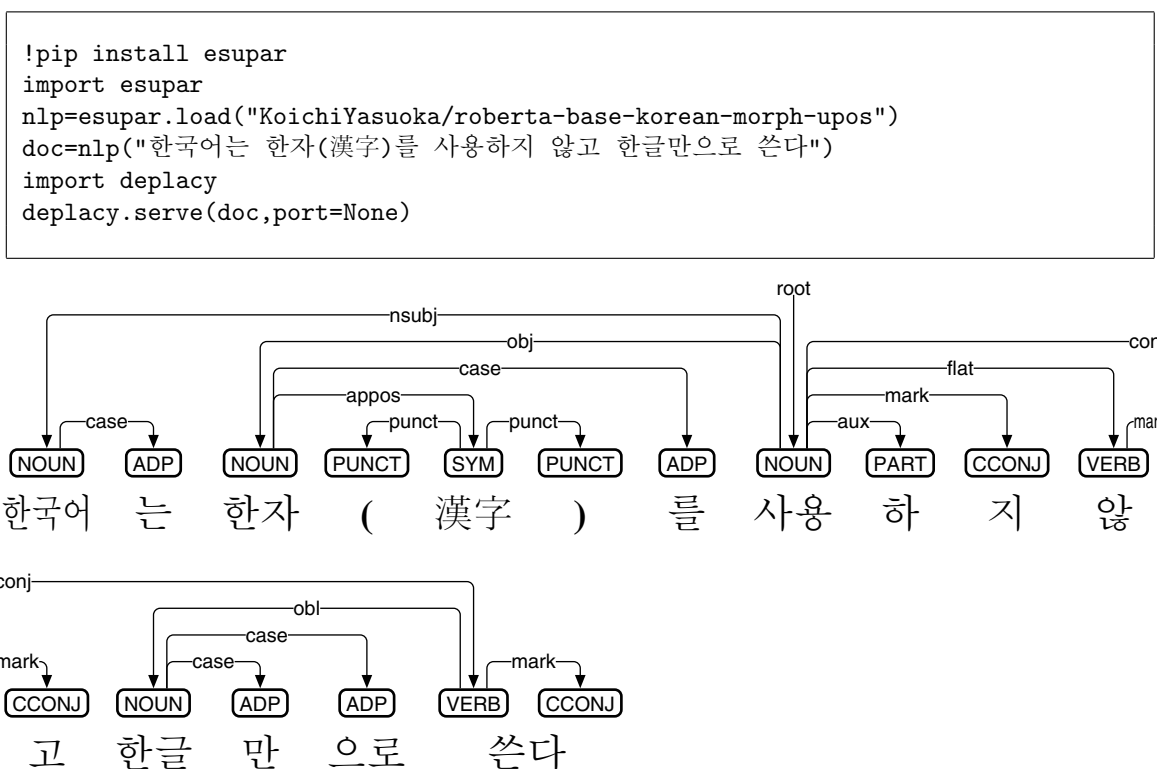
図 167: roberta-base-korean-morph-upos による韓国語の係り受け解析
