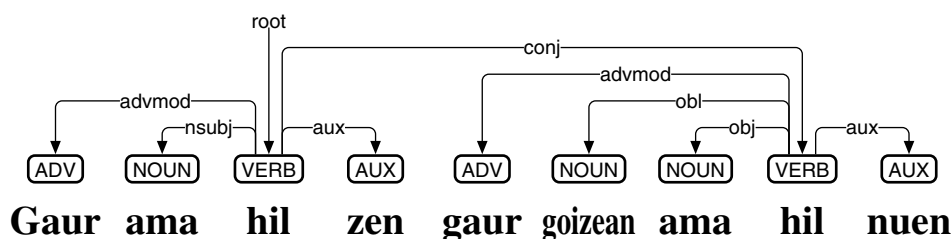
図 159: Trankit によるバスク語の係り受け解析
