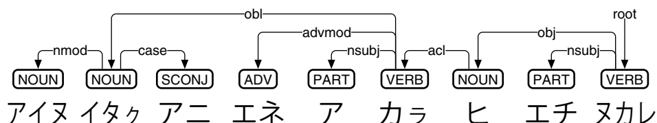
図 181: アイヌ語向け品詞付与・係り受け解析ミニモデルのテスト
