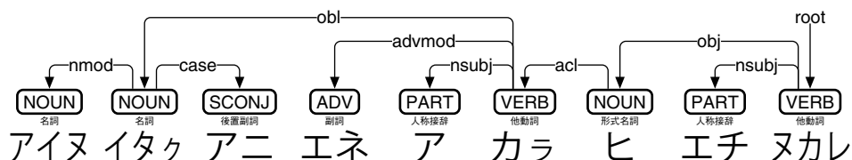
図 173: deberta-base-ainu-upos によるアイヌ語(カタカナ)の係り受け解析
