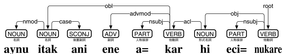
図 174: deberta-base-ainu-upos によるアイヌ語(ラテン文字)の係り受け解析
