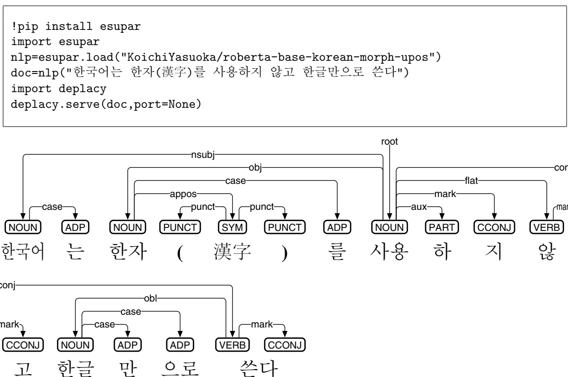
図 161: roberta-base-korean-morph-upos による韓国語の係り受け解析
