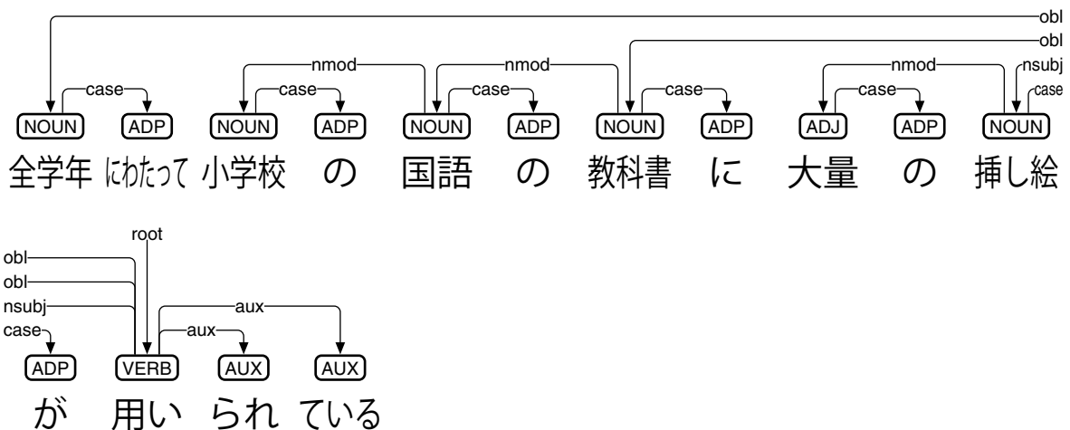
図 34: roberta-base-japanese-luw-upos による日本語係り受け解析 (国語研長単位)
