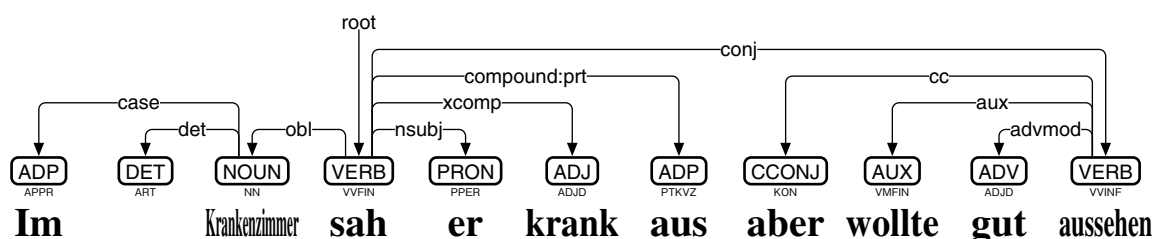
図 54: Trankit によるドイツ語の係り受け解析
