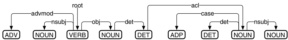
図 98: ベラルーシ語向け品詞付与・係り受け解析ミニモデルのテスト
