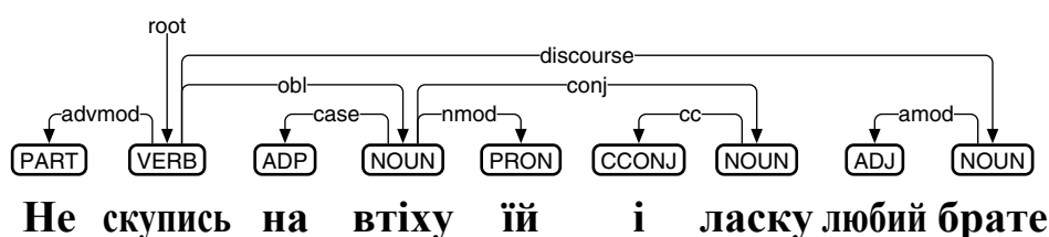
図 81: ウクライナ語向け品詞付与・係り受け解析ミニモデルのテスト
