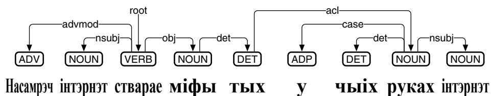
図 87: ベラルーシ語向け品詞付与・係り受け解析ミニモデルのテスト
