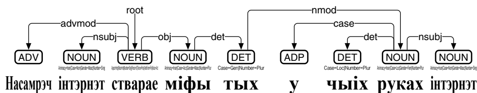
図 82: Camphr-Udify によるベラルーシ語の係り受け解析
