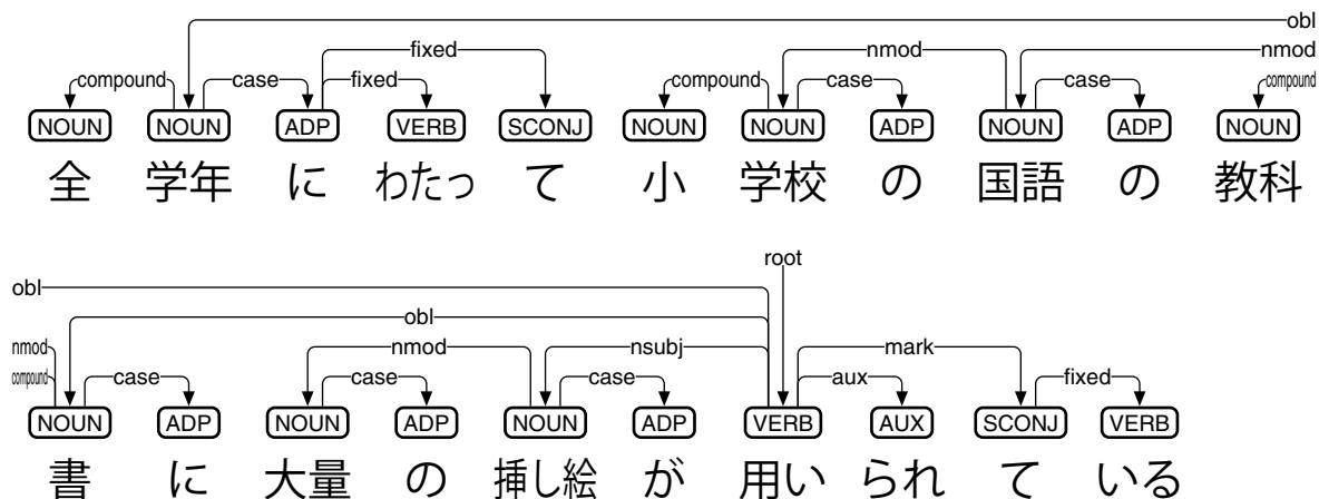
図 29: 国語研短単位向け品詞付与・係り受け解析ミニモデルのテスト
