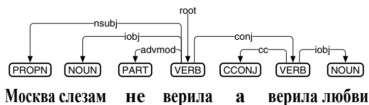
図 70: Trankit によるロシア語の係り受け解析
