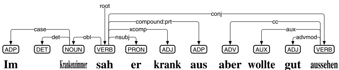
図 55: ドイツ語向け品詞付与・係り受け解析ミニモデルのテスト
