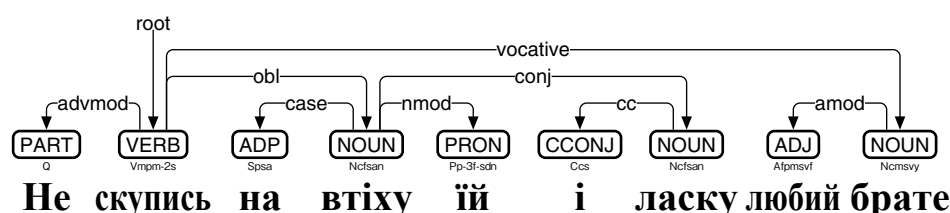
図76: Trankitによるウクライナ語の係り受け解析
