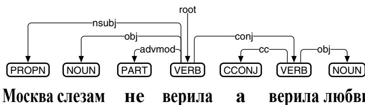
図 75: ロシア語向け品詞付与・係り受け解析ミニモデルのテスト
