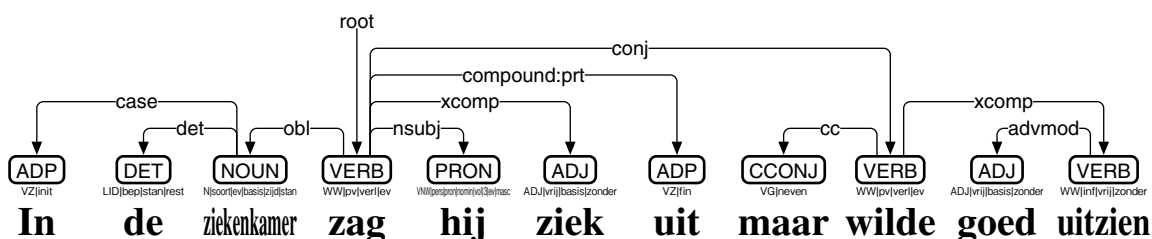
図 57: Trankit によるオランダ語の係り受け解析
