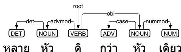
図 64: roberta-base-thai-spm-upos によるタイ語の係り受け解析
