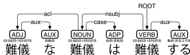
図 24: 国語研短単位 UD における XPOS (UniDic 品詞) と UPOS の関係
