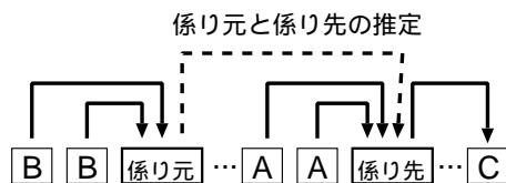
図 3 3つの動的素性
