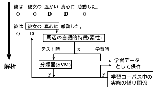
図 2 学習とテストの処理
